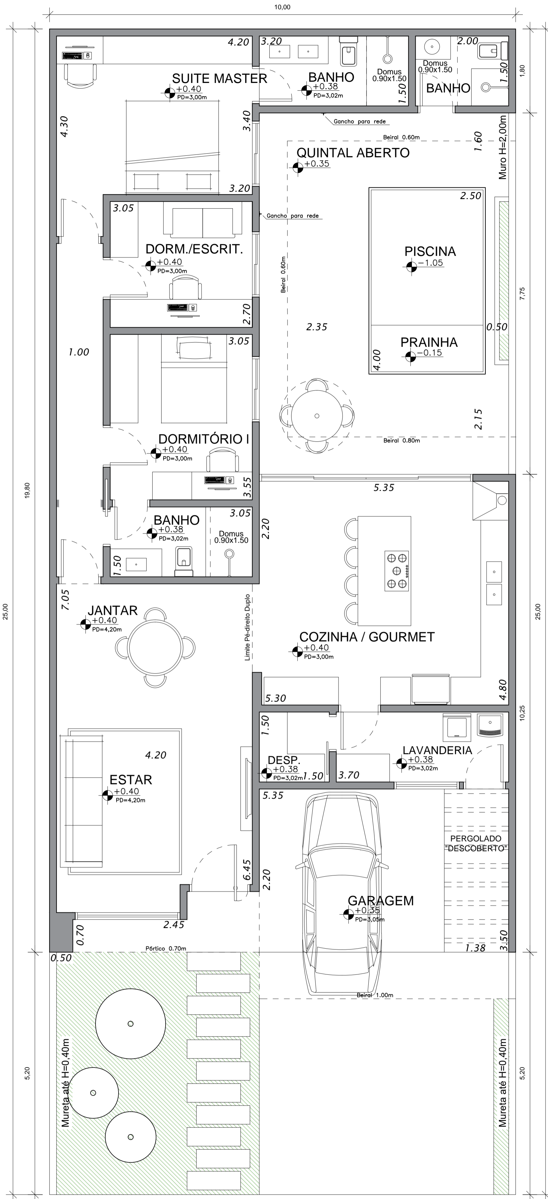
Planta Layout Escala 1:100
