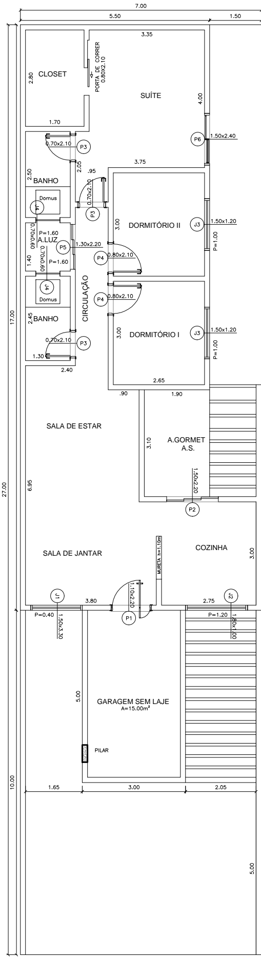
1 PLANTA BAIXA ESCALA 1:100
