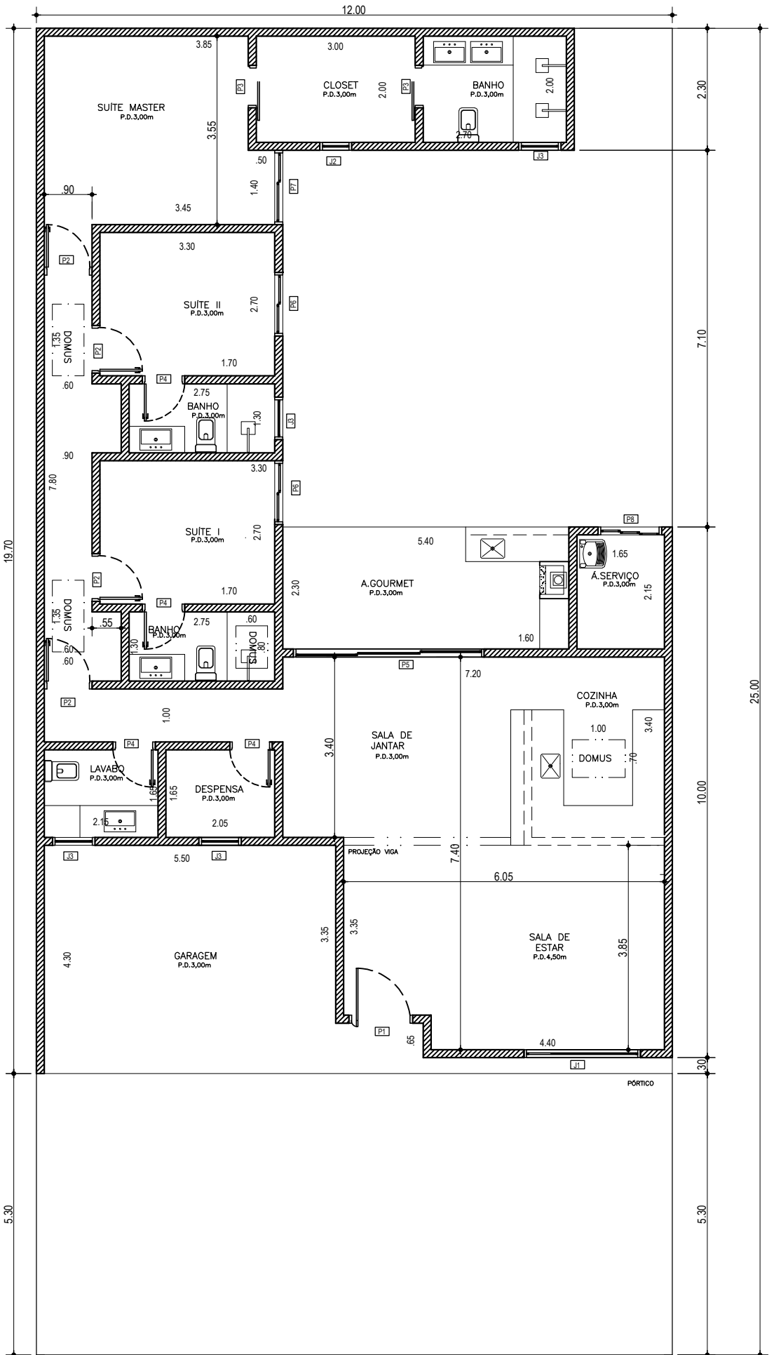
PAVTO. TÉRREO ESC.: 1:100
